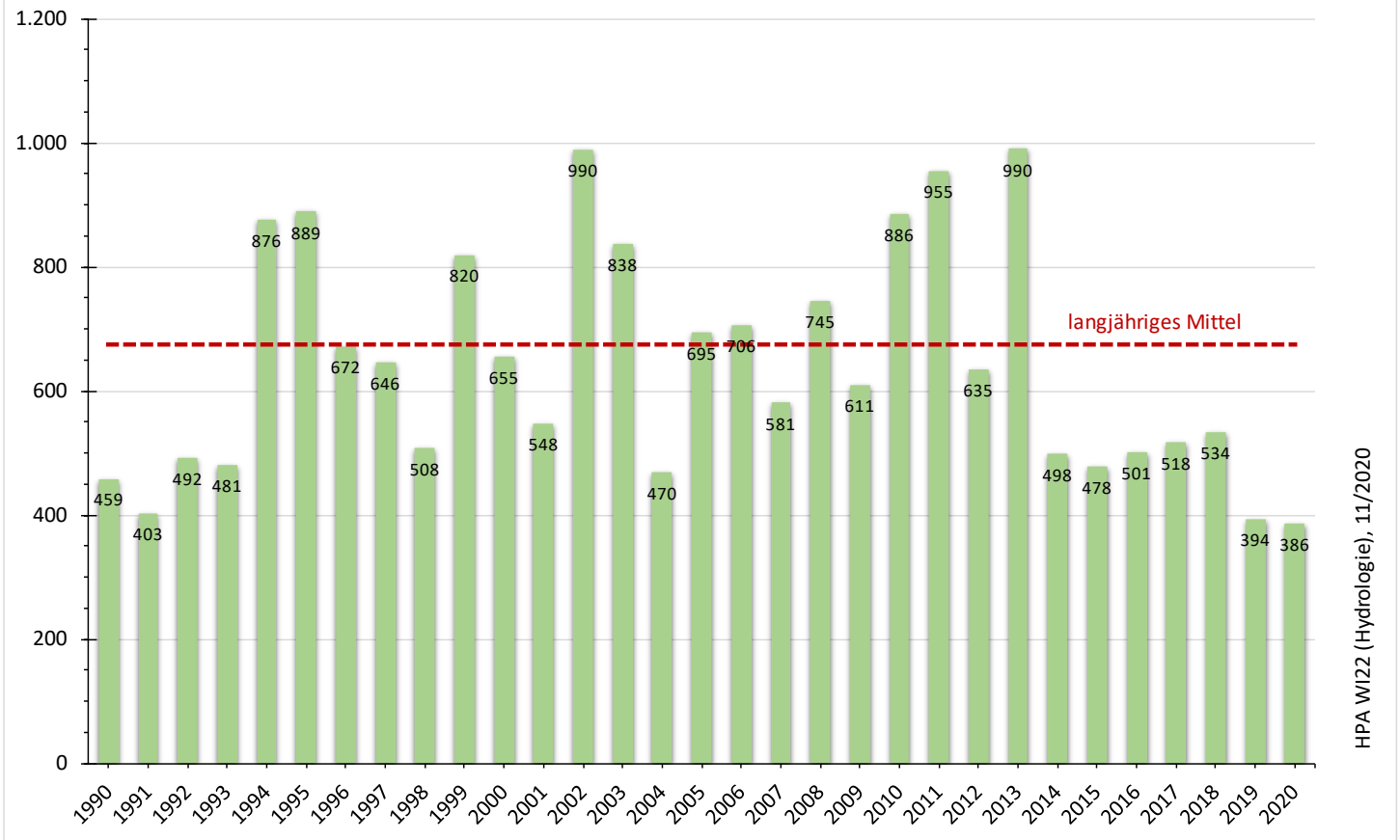
Abfluss Neu Darchau - Jahresmittel seit 1990 (in m 3 /s)
