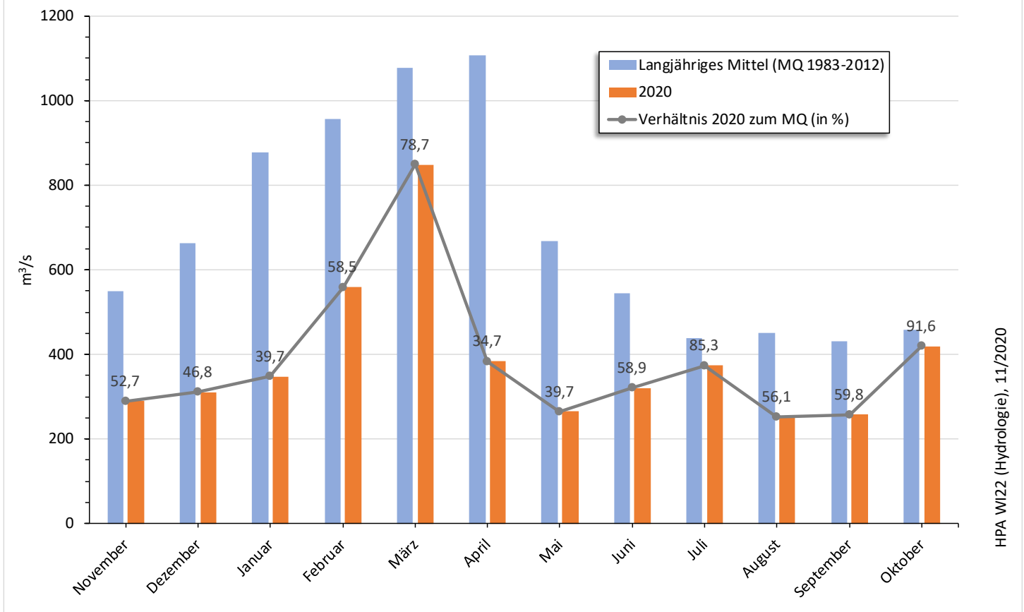
Abfluss Neu Darchau: Monatsmittel 2020 und langjährige Monatsmittel
